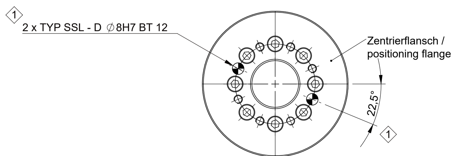
DETAIL D MASSTAB / SCALE 2 : 3
