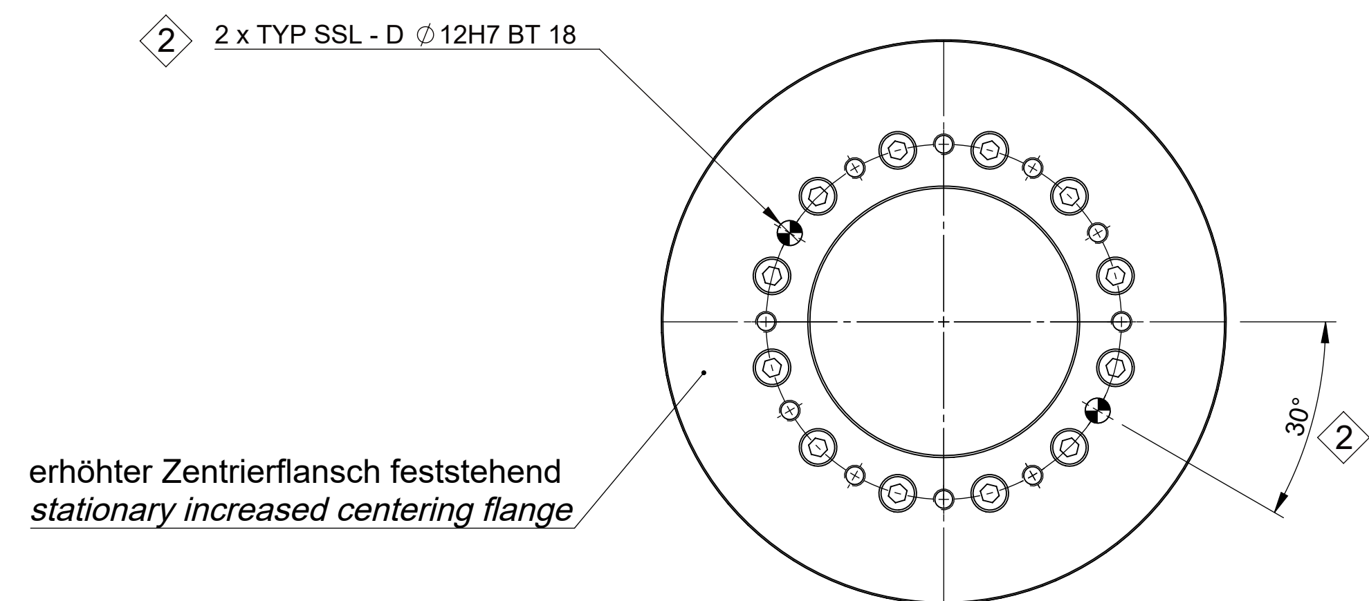
MASSSTAB / SCALE 2 : 5
